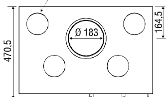
4 sorties Ø125 (uniquement sur modèle I700I)
