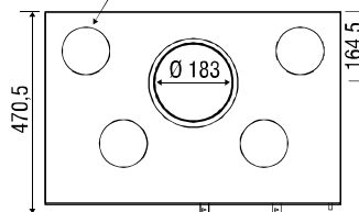
4 sorties Ø125 (uniquement sur modèle I800I)
