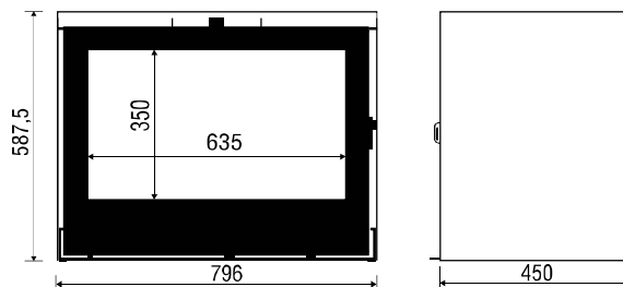
4 sorties Ø125 (uniquement sur modèle I800I)
